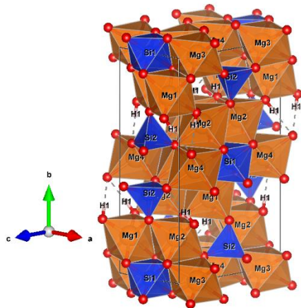
図1 Mg 端成分の superhydrous phase B ( \text{Mg}_{10}\text{Si}_3\text{H}_4\text{O}_{18} ) の結晶構造
