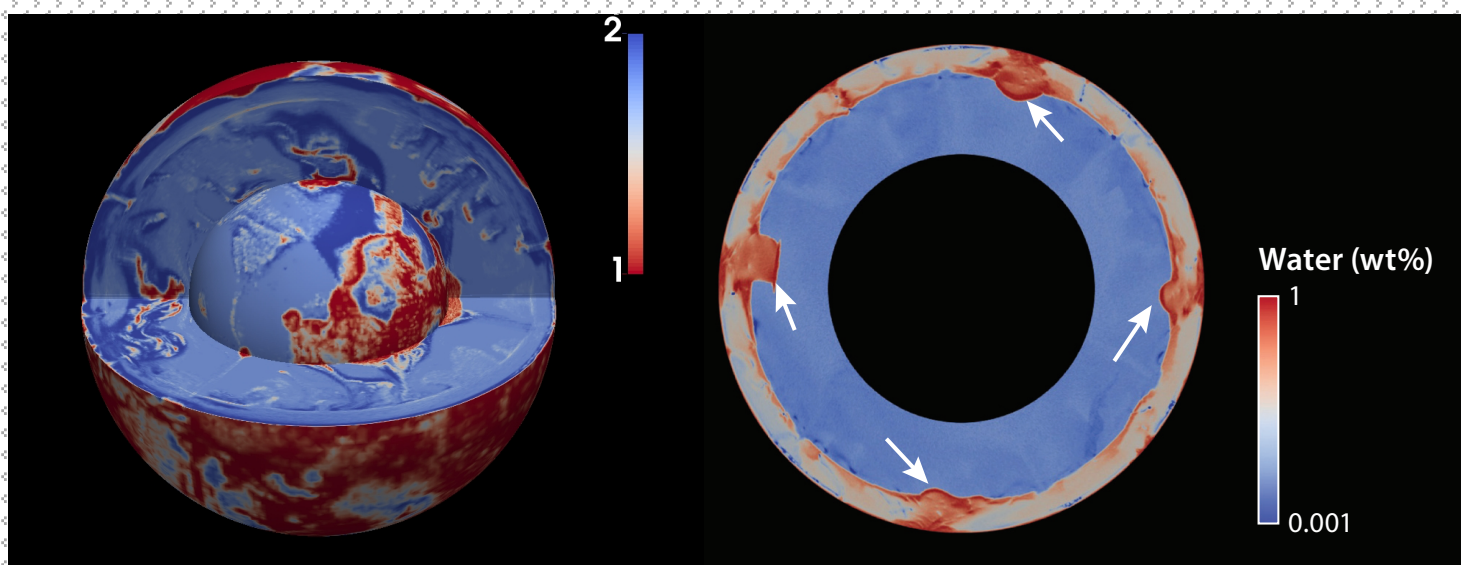
3次元マントル対流シミュレーション 色は組成：赤が玄武岩・青がパイロライト組成
